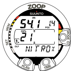
Abb. 3.20 Nitrox-Anzeige. Die maximale Tiefe basierend auf den Einstellungen \text{O}_2 % (21 %) und \text{PO}_2 (1,4 bar) beträgt 54,1 m [177 ft].
