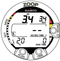
Abb. 3.6 Der Tauchgang hat gerade begonnen.
