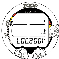
Abb. 4.5 Logbuchoption [1 LOGBOOK].
