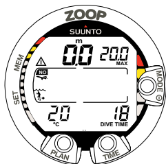
Abb. 3.26 Anzeige im Oberflächenmodus. Sie haben einen 18- minütigen Tauchgang durchgeführt, dessen maximale Tiefe 20,0 m [66 ft] betrug. Ihre aktuelle Tiefe ist 0,0 m [0 ft]. Das Flugverbots-Symbol zeigt, dass Sie nicht fliegen sollten und das ACHTUNG-Symbol weist Sie darauf hin, dass Sie Ihre Oberflächenpause wegen des Auftretens von Mikrobläschen verlängern sollten.
