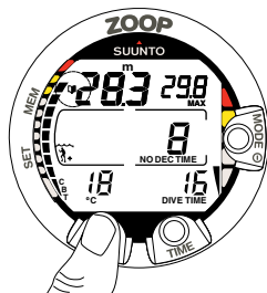
Abb. 3.8 Hinterlegen eines Lesezeichens. Ein Lesezeichen wird im Profilspeicher während des Tauchgangs eingetragen, indem der PLAN-Kontakt gedrückt wird. Beachten Sie das Logbuchsymbol, links neben der Tiefe.
