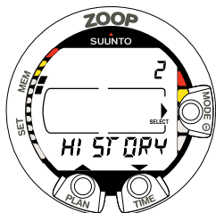
Abb. 4.12 Untermenü Tauchgangs-Historie. [2 HISTORY].
