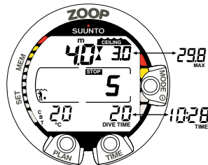
Abb. 3.13 Verbindlicher Sicherheitsstopp. Sie werden aufgefordert, einen verbindlichen Sicherheitsstopp in einem Tiefenbereich zwischen 6 m und 3 m [20 ft - 10 ft] durchzuführen. Durch Drücken von TIME erscheint die alternative Anzeige.
