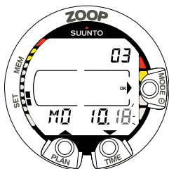
Abb. 4.23 Einstellen des Datums.
