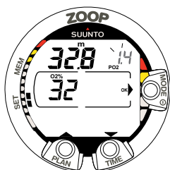
Abb. 4.17 Einstellen des Sauerstoff-Prozentsatzes und Teildrucks. Die zugehörige maximale Tiefe ist 32,8 m [107 ft]. Drücken Sie PLAN und TIME, um den Sauerstoff-Prozentsatz zu ändern und den Sauerstoff-Teildruck einzustellen.
