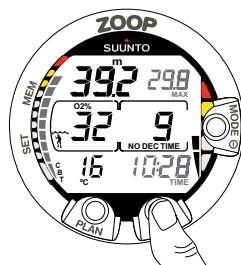
Abb. 3.24 Alternative Anzeige. Nach Drücken des TIME-Kontakts werden die aktuelle Uhrzeit, die maximale Tiefe, Wassertemperatur, CBT und O_2 % angezeigt.
