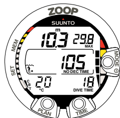
Abb. 3.11. Aufstiegs-geschwindigkeitsanzeige: Maximal erlaubte Aufstiegsgeschwindigkeit. 4 Segmente.
