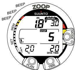
Abb. 3.14 Nicht eingehaltener verbindlicher Sicherheitsstopp. Ein abwärts gerichteter Pfeil und ein akustischer Alarm signalisieren, dass Sie auf die für den Sicherheitsstopp vorgegebene Tiefe abtauchen sollen.
