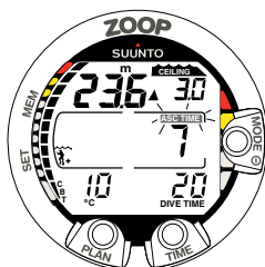
Abb. 3.15 Dekompressionsstauchgang unterhalb der Dekompressionsgrenze. Der aufwärts gerichtete Pfeil und die blinkende Anzeige ASC TIME weisen Sie darauf hin, aufzusteigen. Die minimale Aufstiegszeit beinhaltet den Sicherheitsstopp und beträgt 7 Minuten. Die Deko-Stufe liegt bei 3 m [10 ft].
