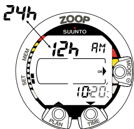
Abb. 4.22 Einstellen der Uhrzeit.
