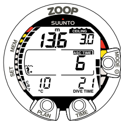
Abb. 3.16 Dekompressionsstauchgang oberhalb der Dekompressionsgrenze. Der aufwärts gerichtete Pfeil ist verschwunden und ASC TIME blinkt nicht mehr, d.h. Sie befinden sich im Dekompressionsbereich.
