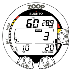
Abb. 3.9 3-minütiger empfohlener Sicherheitsstopp.
