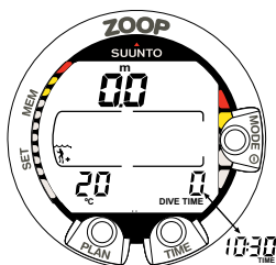
Abb. 3.3 Aktivierung III. Oberflächenmodus: Tiefe und Tauchzeit sind Null, die Temperatur beträgt 20°C. Durch Betätigen des TIME Kontakts können Sie die Anzeige von aktueller Uhrzeit oder des alternativen Displays aktivieren.
