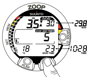
Abb. 3.17 Dekompressions-tauchgang innerhalb der Dekompressionszone. Zwei gegeneinander gerichtete Pfeile (Sanduhr) erscheinen. Sie befinden sich im optimalen Deko-Bereich in 3,5 m [11 ft] Tiefe und Ihre minimale Aufstiegszeit beträgt 5 Minuten. Durch Drücken des TIME-Kontaktes können Sie die maximale Tiefe, Uhrzeit und Temperatur ablesen.
