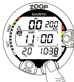
Abb. 3.28 Oberflächenintervall, Flugwarnung. Ein zweimaliges Drücken des TIME-Kontaktes zeigt die Zeit bis zum Ablauf der Flugverbotszeit an, symbolisiert durch ein Flugzeug.
