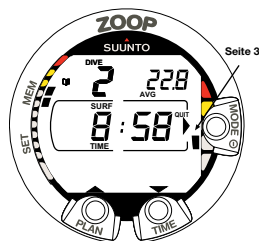
Abb. 4.8 Logbuch, Seite III. Oberflächenintervall und durchschnittliche Tiefe.
