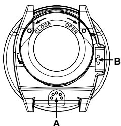
Abb. 2.3 Tiefensensor (A), Wasserkontakte/Datenüber- tragungskontakte (B).
