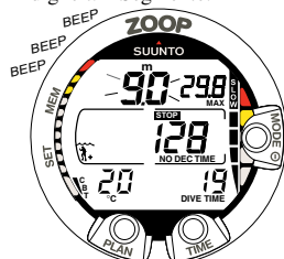
Abb. 3.12 Aufstiegsgeschwindigkeitsanzeige. Blinkende Tiefenanzeige. SLOW und 4 Segmente werden angezeigt mit einem akustischen Alarm: Aufstiegsgeschwindigkeit liegt über 10 m/Min [33 ft/min]. Dies ist ein Hinweis, die Geschwindigkeit zu reduzieren. Das STOP-Symbol erscheint, weil Sie einen vorgegebenen Sicherheitsstopp in einer Tiefe von 6 m durchführen sollten.
