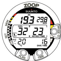
Abb. 3.22 Tauchen im Nitrox-Modus. \text{O}_2 % ist auf 32 % eingestellt.
