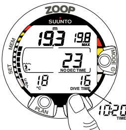
Abb. 3.7 Anzeige während des Tauchgangs. Die aktuelle Tiefe ist 19,3 m und die Nullzeit beträgt im Modus A0/P1 23 Minuten. Die maximal bei diesem Tauchgang erreichte Tiefe war 19,8 m, bisherige Tauchzeit ist 16 Minuten und die Wassertemperatur beträgt 18°C [64°F]. Nach Drücken des TIME-Kontakts wird die aktuelle Uhrzeit 10:20 [10:20 am] für 5 Sekunden angezeigt.
