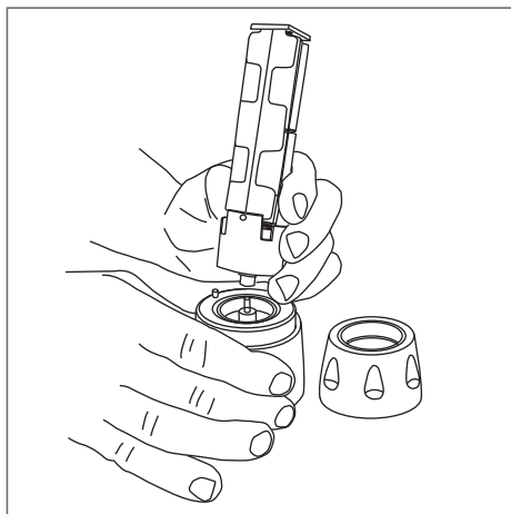
Zeichnung 8 - Richtiges Einsetzen des Batteriebehälters
