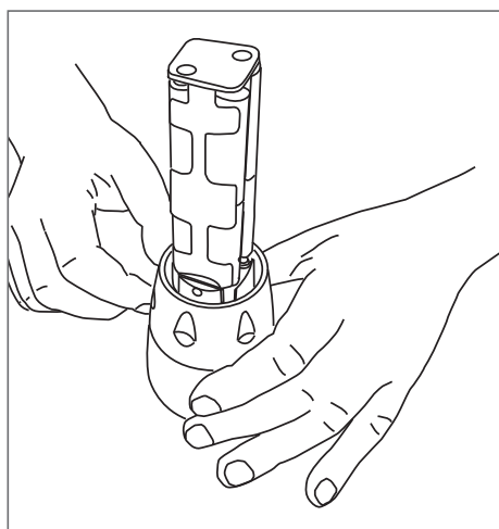
Zeichnung 11 - Funktionskontrolle der Schaltvorrichtung
