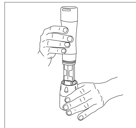
Zeichnung 12 - Aufsetzen des Lampengehäuses auf den Batteriebehälter
