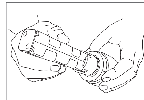
Dis. 9 - Colocación del cesto porta-baterías en el grupo ventanilla (cabeza de la linterna)
