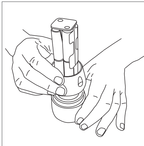
Dessin 10 - Mise en place de la bague d'allumage
