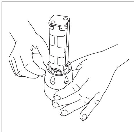
Dessin 11 - Contrôle du bon fonctionnement de la bague d'allumage
