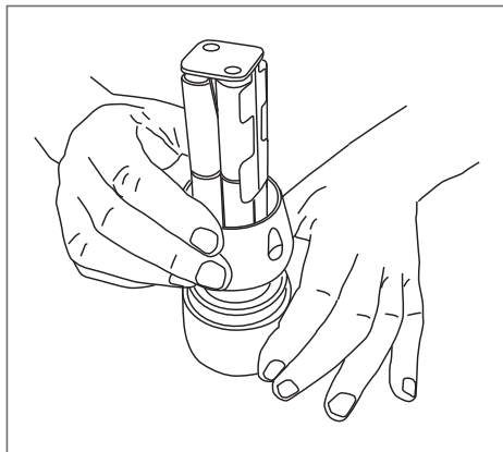
Fig. 10 - Corretto inserimento della ghiera d'accensione
