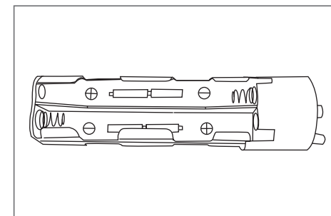
Zeichnung 6 - Abbildung der elektrischen Pole auf dem Batteriebehälter
