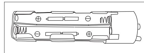
Fig. 6 - Illustrazione delle polarità poste sul cestello porta batterie
