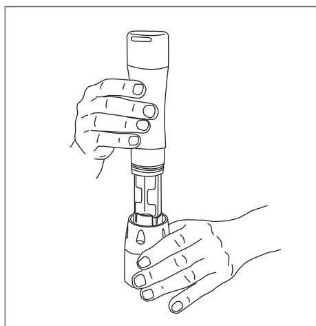
Fig. 12 - Inserimento del corpo torcia sul cestello porta batterie
