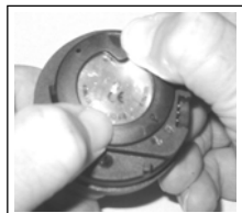
Fig. 69 - EINSETZEN DES HALTERINGS
