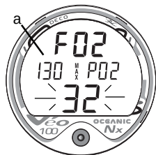
Fig. 19 - FO2 EINSTELLUNG 32% (MOD 40M/130FT)
