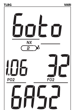
Abb. 60 - GAS WECHSEL-VORSCHAU
