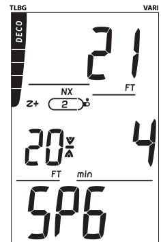
Abb. 63 - DEKOSTOPP HAUPT
