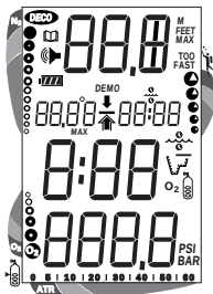
Abb. 14 - Selbsttest-Modus
