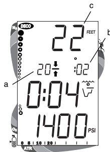
Abb. 56 - Dekompression, Anzeige #1
