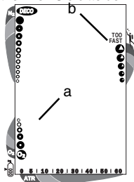
Abb. 3 - Balkenanzeige O 2 und Aufstiegsgeschwindigkeit
