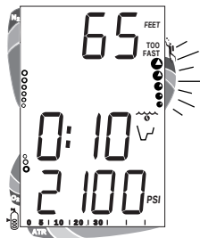
Abb. 47 - Aufstiegsalarm
